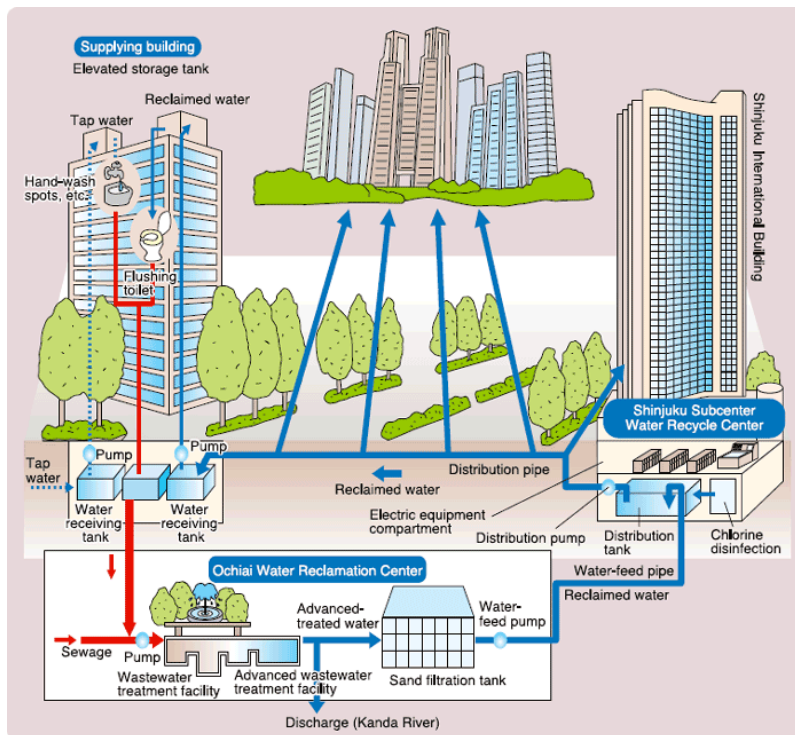
Abb.7: Brauchwasser-Aufbereitung und Wiederverwendung in Tokio (Quelle: www.gesui.metro.tokyo )
