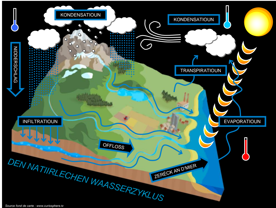
Abb. 1 : Der Wasserkreislauf (Quelle: Pfister/CRP (L)/ www.curiosphere.tv)
